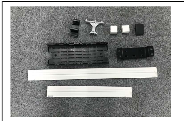
4 配線トレー 8個/中央 配線カバー16個 (W3000用x8 W2000用x8)/配線カバー受け 16個/配線カバー脇エンドキャップ 16個、センターエンドキャップx8個/配線カバー受け部材x32個/コードカバー受け部材x4個
